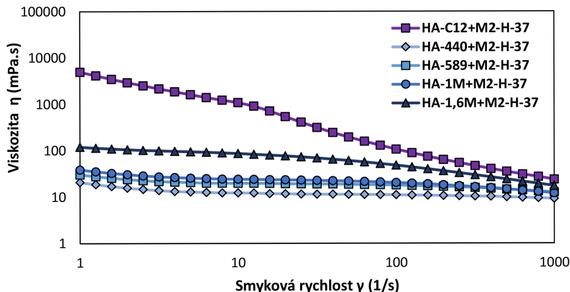
Obr. 5-8 Viskozitní charakteristika vzorků KH po interakci s M2 v H-pufru.
