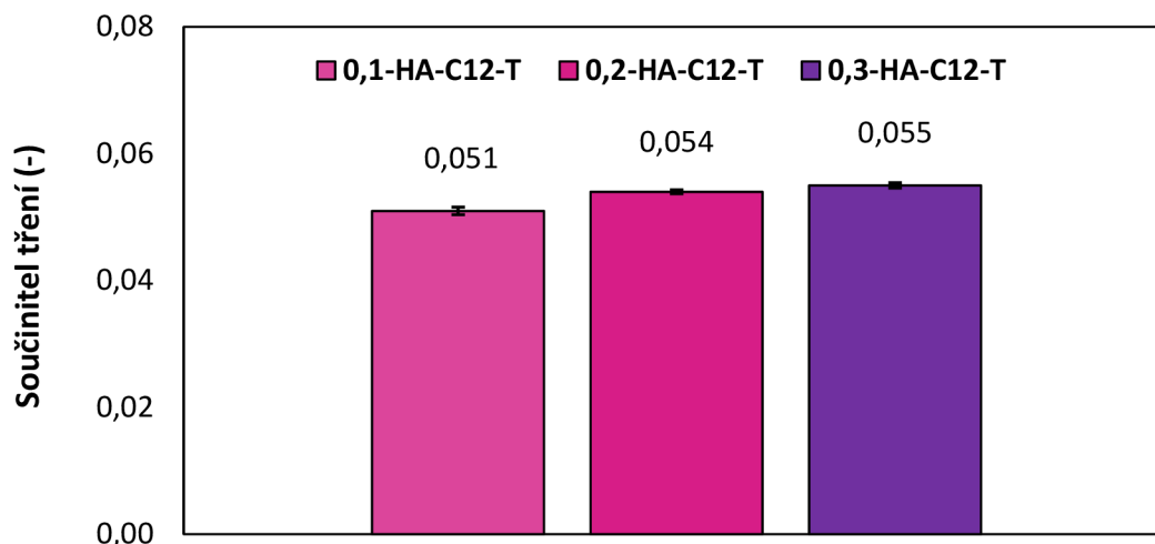
Obr. 5-20 Graf zobrazující změnu součinitele tření derivátu v závislosti na koncentraci polymeru (T-pufry).
