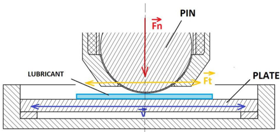
Obr. 4-10 Konfigurace pin-on-plate.
