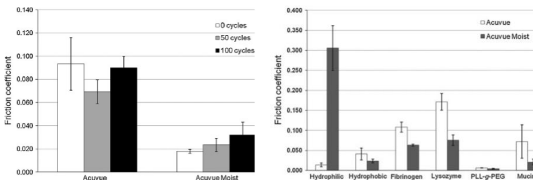
Obr. 2-14 Vliv počtu zátěžných cyklů na součinitel tření (a), vliv povrchové úpravy skleněného protikusu na součinitel tření (b) [26].
