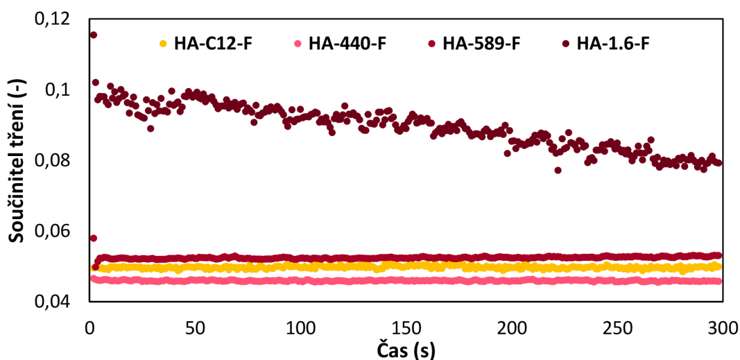
Obr. 5-16 Vývoj součinitele tření v závislosti na čase pro vzorky v F-pufru.
