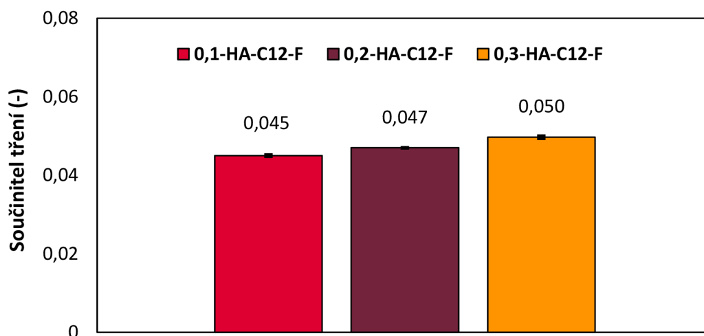
Obr. 5-21 Graf zobrazující změnu součinitele tření derivátu v závislosti na koncentraci polymeru (F-pufry).
