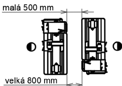
Obr. 17 Stroje zadními stranami k sobě. [5]
