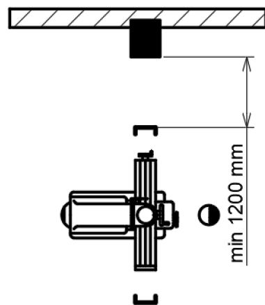
Obr. 28 Stroj s pohyblivou částí směřující ke stěně. [5]
