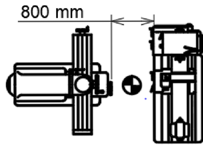
Obr. 20 Stroje čelními stranami k sobě, obsluha dvou strojů. [5]
