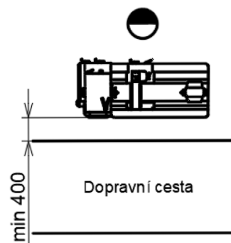
Obr. 24 Stroj zadní stranou k cestě. [5]
