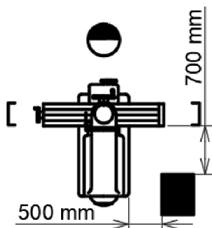
Obr. 29 Stroj s boční a zadní stranou u sloupu. [5]
