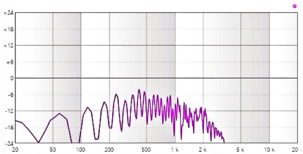
B2: Modulová kmitočtová charakteristika spektra tónu B 1 s odrazem od zdi (lesnice, nátrubek V. Bach 10)
