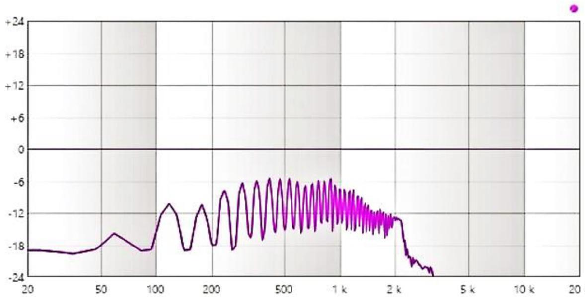
B1: Modulová kmitočtová charakteristika spektra tónu B 1 (lesnice, nátrubek V. Bach 10)
