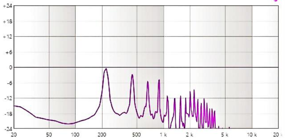
B4: Modulová kmitočtová charakteristika spektra tónu a s odrazem od zdi (lesnice, nátrubek V. Bach 10)
