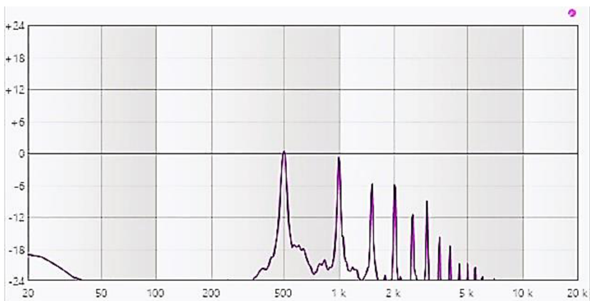
A6: Modulová kmitočtová charakteristika spektra tónu h^1 s odrazem od zdi (f hmaty, nátrubek V. Bach 10)
