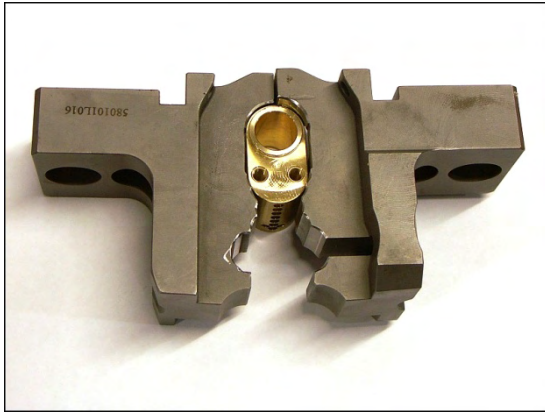
Upnutí tělesa typu ovál.
