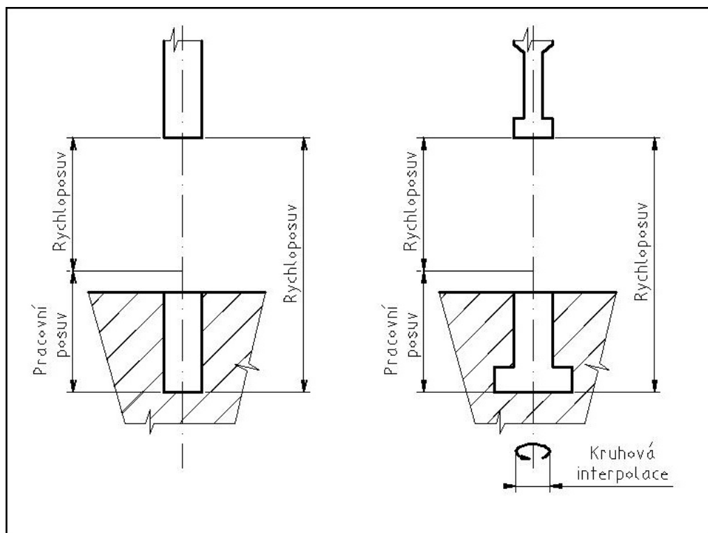
Obr. 5.7. Schéma dráhy nástroje.
