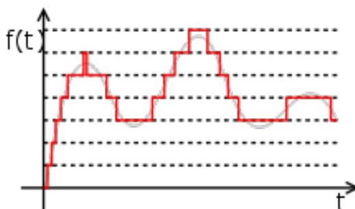
Obr. 1.5: Kvantizace signálu
