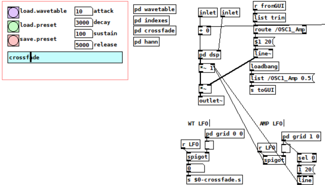
Obr. 3.12: Wavetable oscilátor
