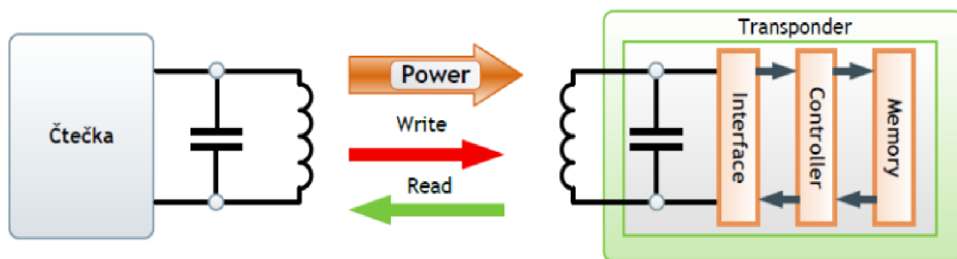
Obr. 1.1 Základní schéma komunikace v RFID
