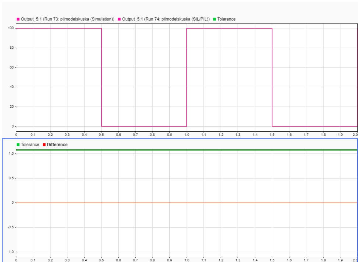
Obr. 16: Výstupné porovnanie signálov PIL simulácie
