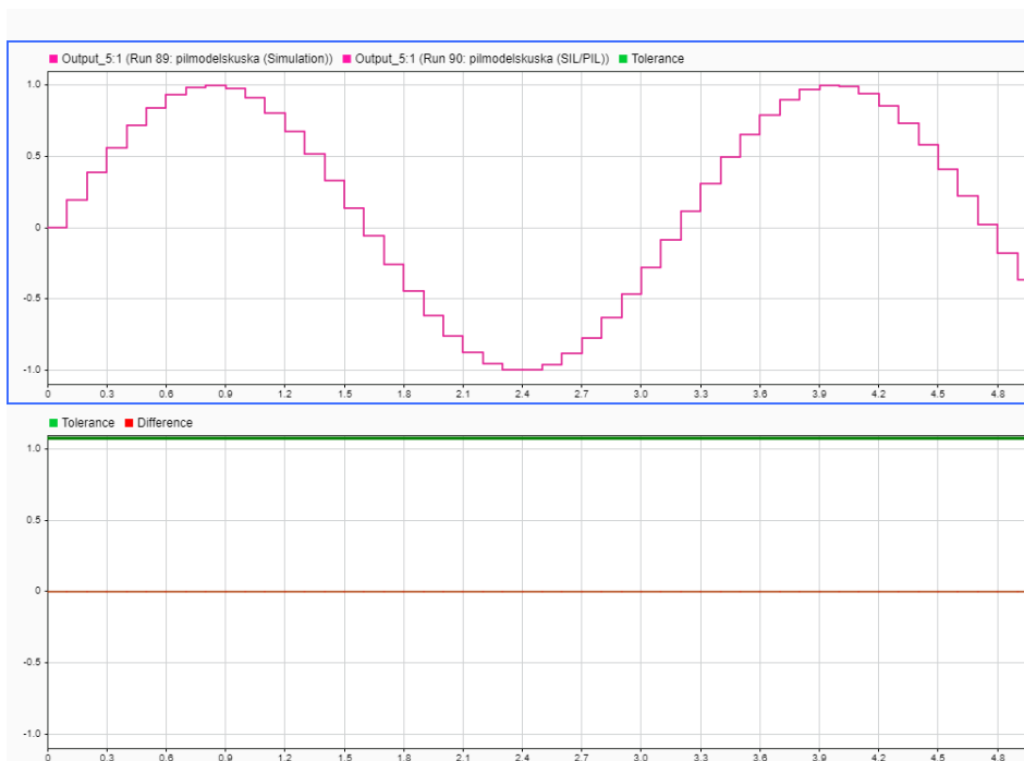
Obr. 19: Výstupné porovnanie signálov PIL simulácie
