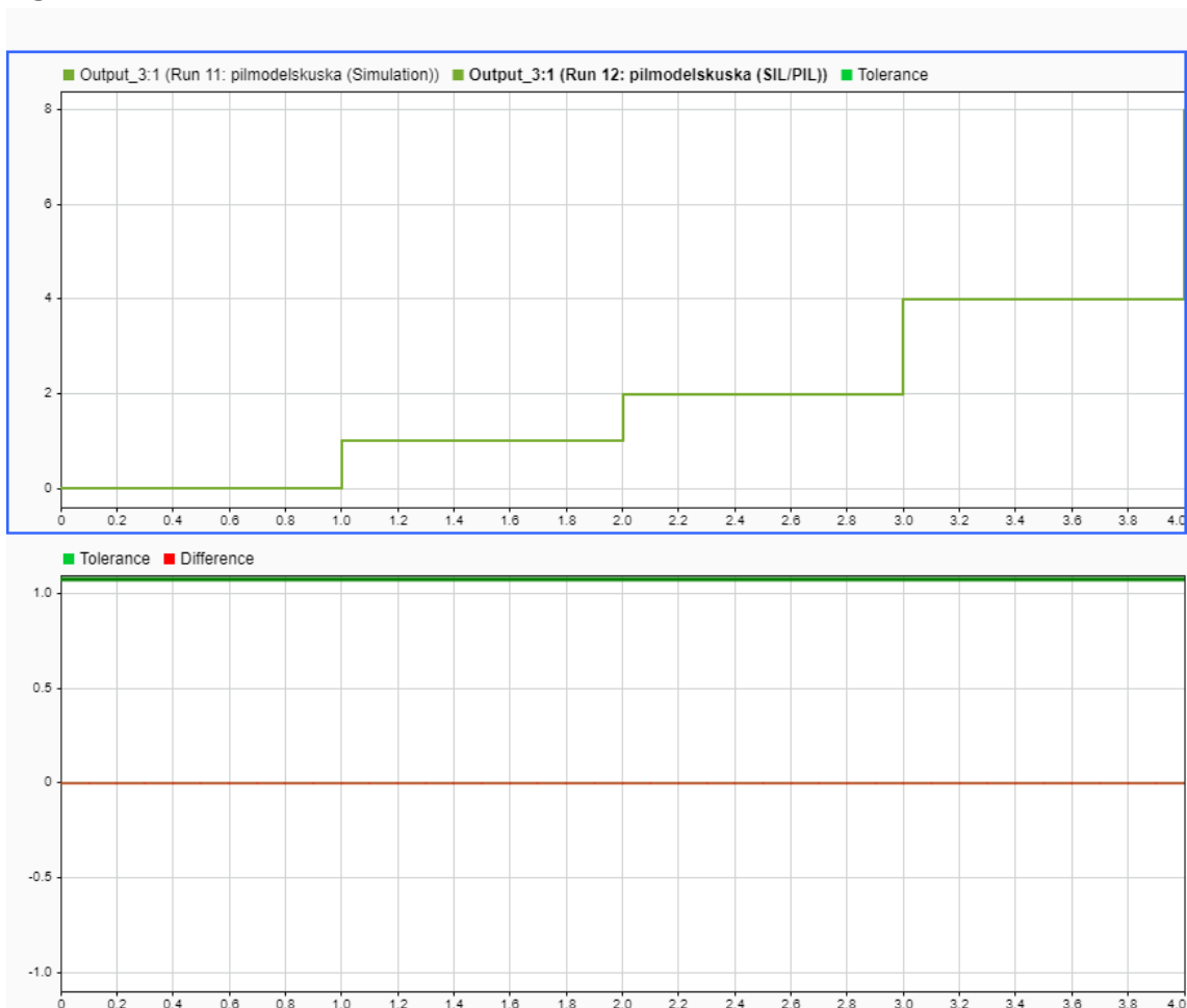
Obr. 12: Výstupné porovnanie signálov SIL simulácie
