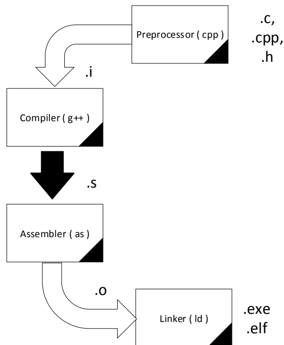
Obr. 6: Znáozornenie procesu kompilácie [25]
