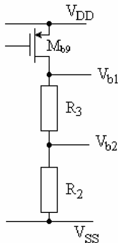
Obr. 23 Dělič napětí
