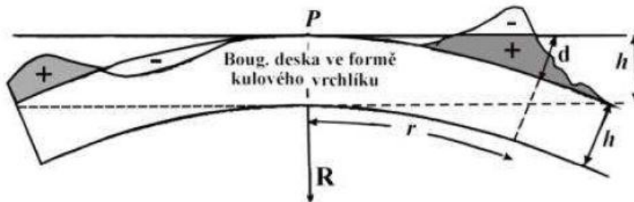
Obrázok č. 19 Schéma predstavujúca vplyv topografických hmôt [23]
