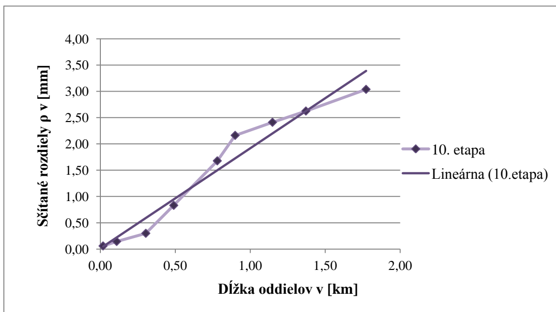
Graf č. 1 Vplyv systematických chýb
