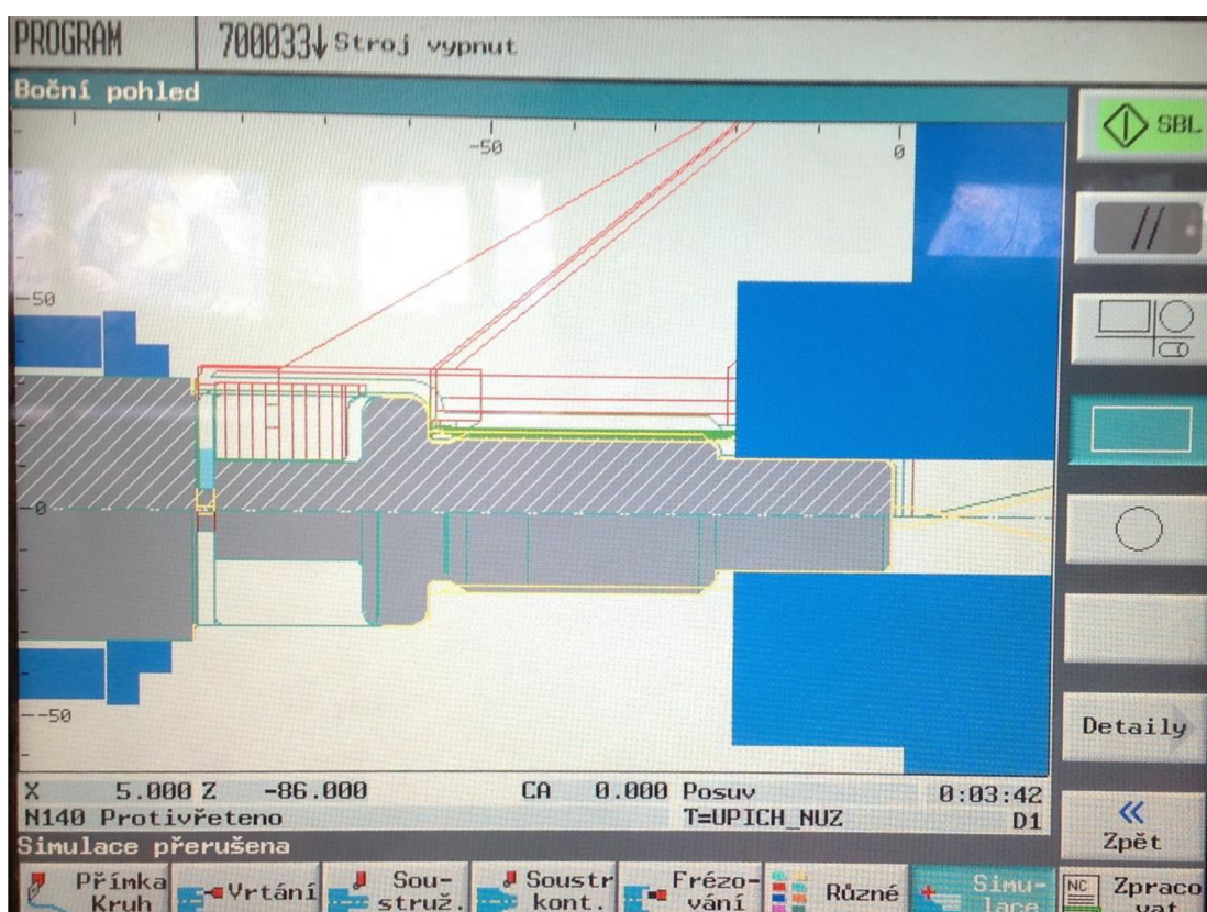
Obr. 30 Cyklus upichování.
