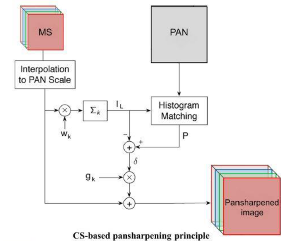
Obr. 2: Princip pansharpeneru založený na metodě CS (Yilmaz a kol., 2022).
