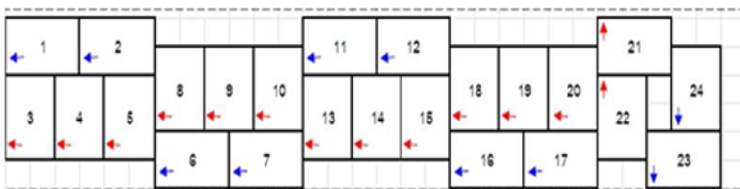
Obr. 3.2 Maximální využití kontejneru 40' GP (24 palet ve 2 vrstvách)
