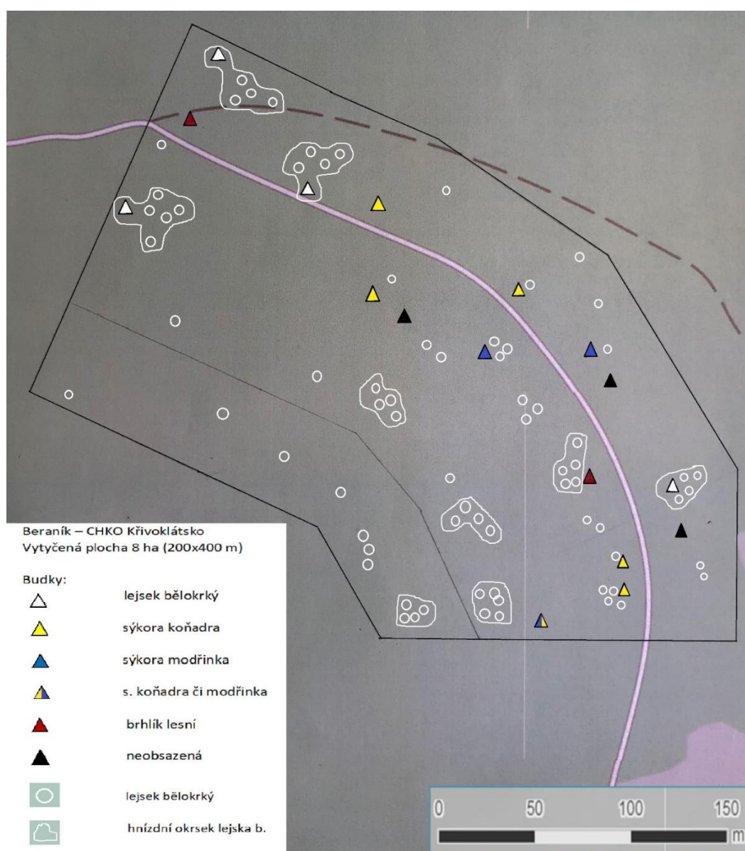
Obrázek 37: Druhová mapa lejska bělokrkého
