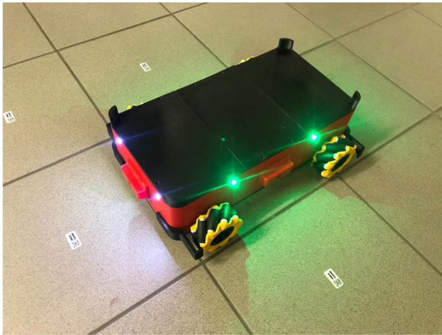
Obrázek 7.4 Výsledná realizace voztítko
