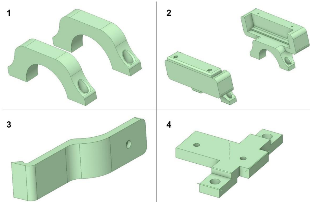
Obrázek 2.7 Doplňkové díly pro realizaci voztka
