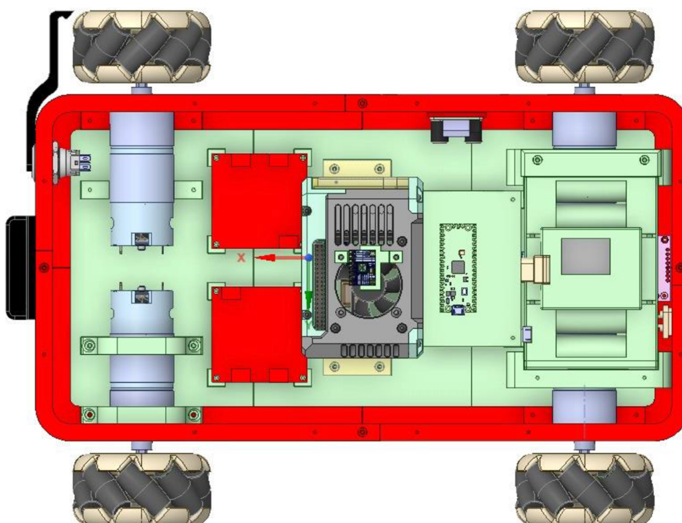
Obrázek 2.9 Rozmístění komponentů
