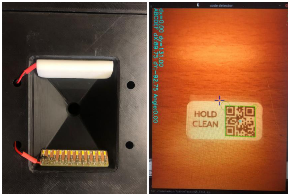
Obrázek 4.13 Snímek z kamery – LED pásek
