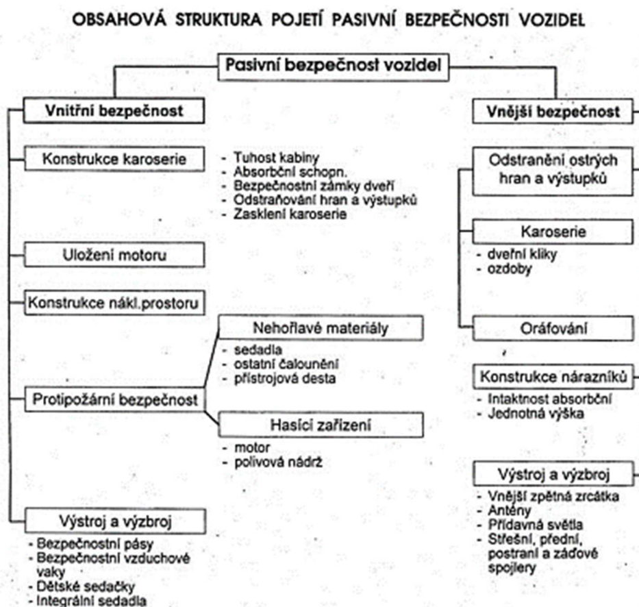
Obrázek č. 2 - Schéma pasivní bezpečnosti vozidla 14
