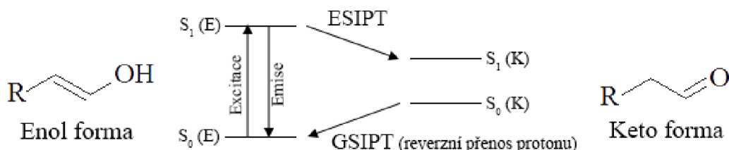
Obr. 12 Mechanismus ESIPT
