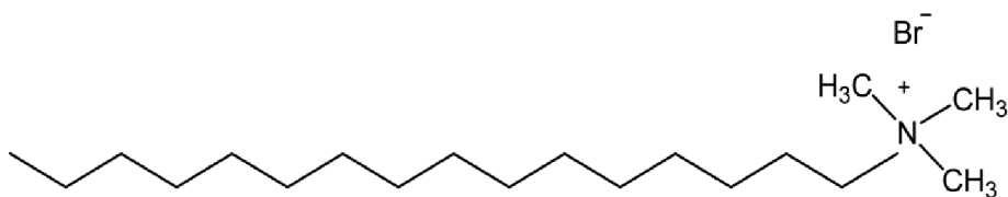
Obr. 3 Kationtový tenzid – CTAB
