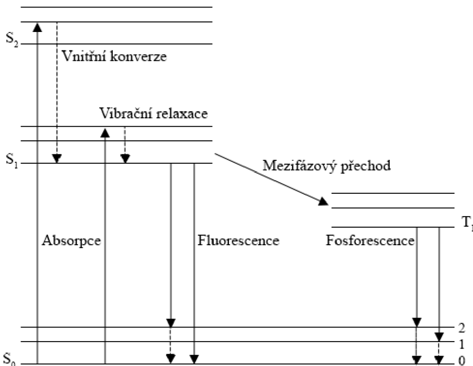
Obr. 9 Jablonského diagram
