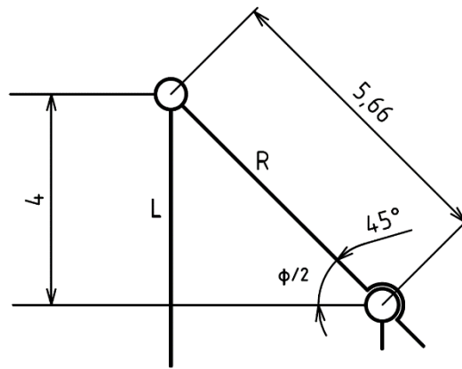
Obr. 14: Výpočtový trojúhelník
