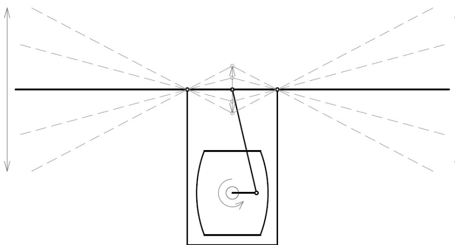
Obr. 13: Navržené kinematické ústrojí
