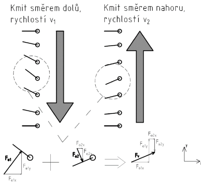
Obr. 15: Síla způsobená rozdílnou rychlostí kmitů
