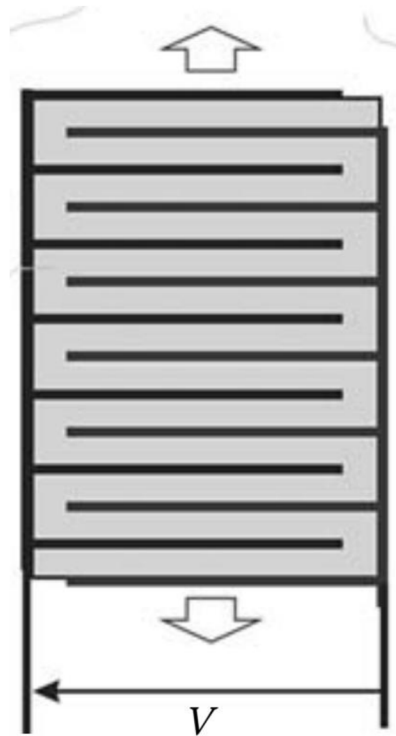
Obr. 6: Sendvičově naskládané piezoaktuátory
