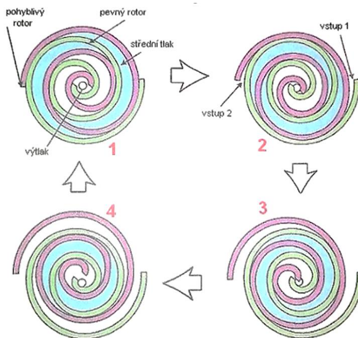
Obrázek 15 Pohyb kompresoru Scroll [4]
