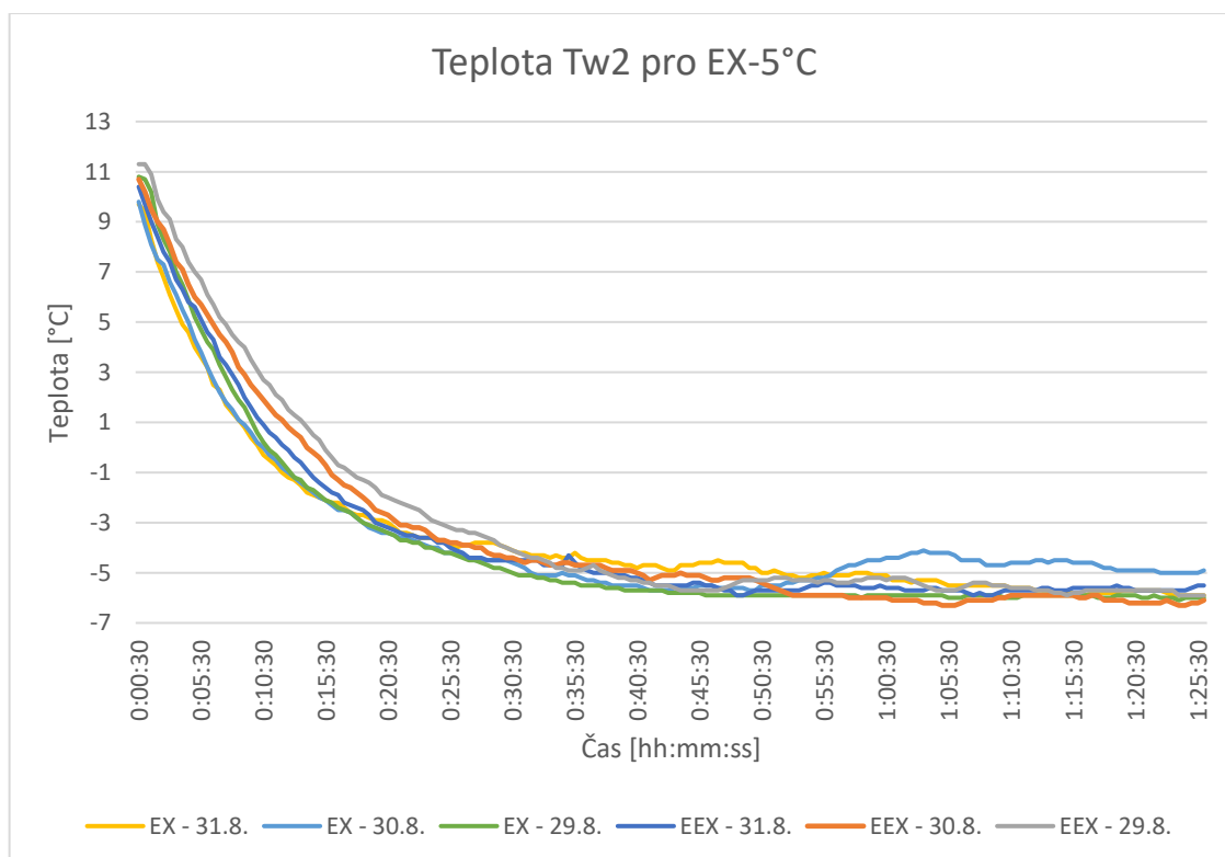
Graf 5 Porovnání průměrných hodnot pro referenční teplotu -5 °C
