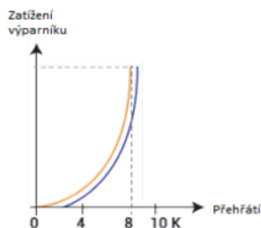
Obrázek 24 Chování elektrického expanzního ventilu [6]
