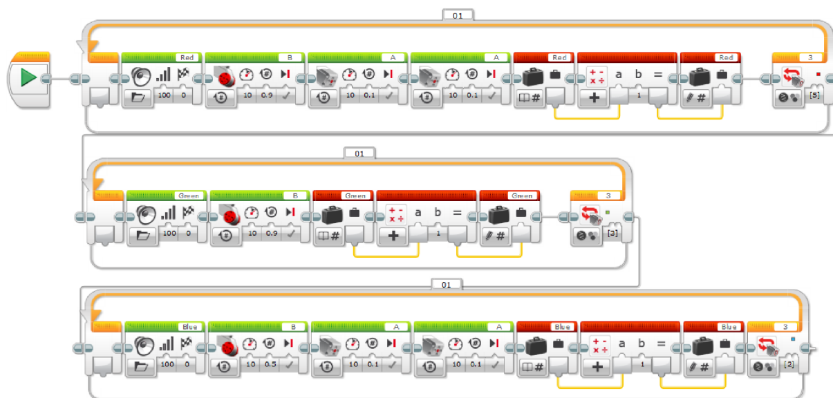
Obrázek 33: Vytvořený blok pro roztřídění barev
