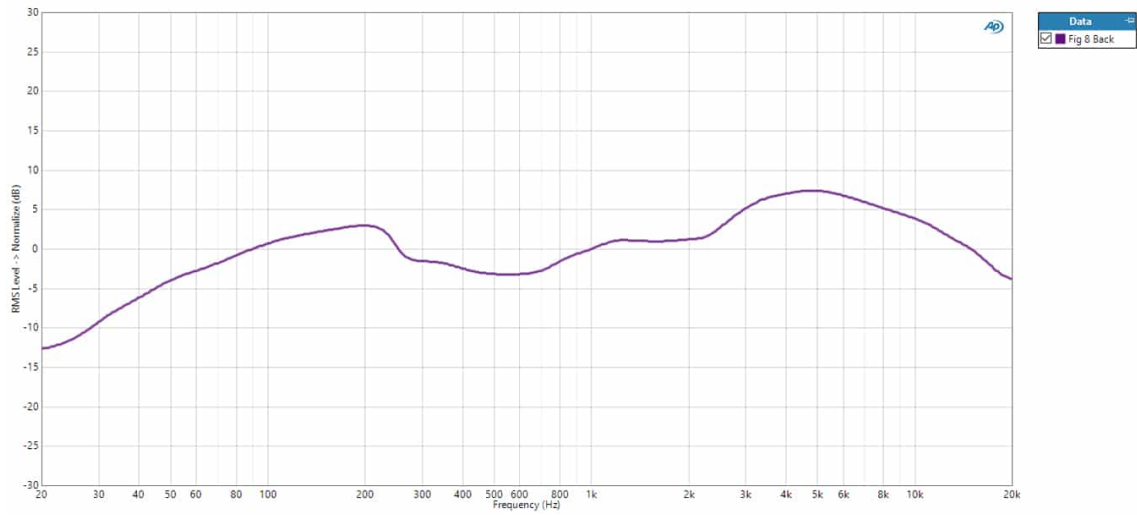
Obr. A.3: Osmičková charakteristika - zadní strana
