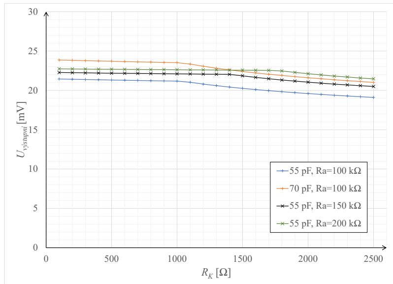
Obr. 3.4: Graf závislosti výstupního napětí na velikosti katodového odporu pro různé hodnoty anodového odporu
