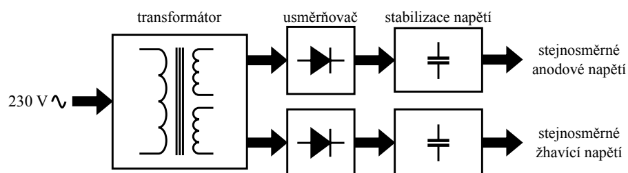
Obr. 1.9: Blokové schéma napájení pro elektronkový mikrofon
