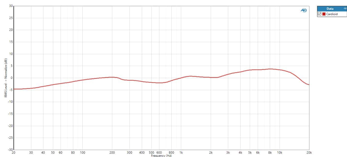
Obr. A.1: Kardiodní charakteristika - přední strana
