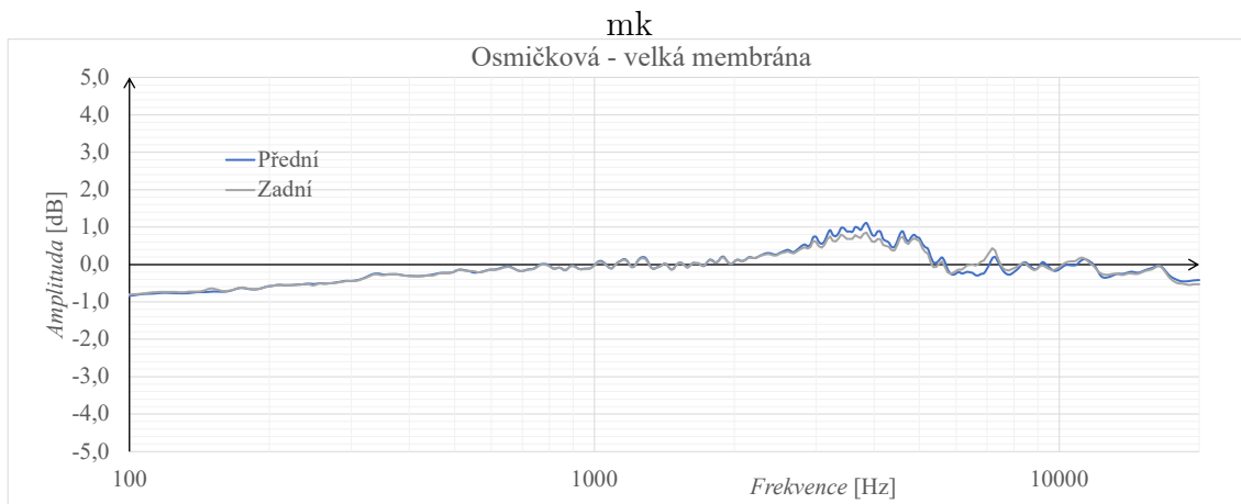
Obr. 5.5: Graf kmitočtové charakteristiky - osmičková, velká membrána
