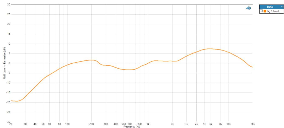
Obr. A.2: Osmičková charakteristika - přední strana
