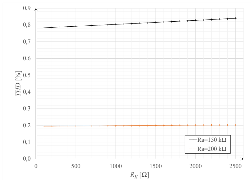
Obr. 3.5: Graf závislosti THD na velikosti katodového odporu pro různé hodnoty anodového odporu
