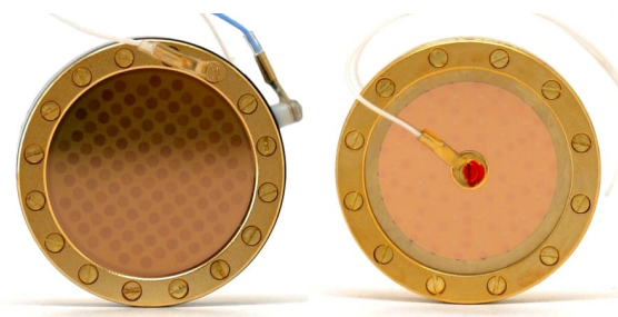
Obr. 1.3: Vpravo kapsle s kontaktem na přitlačném kroužku, vlevo s kontaktem uprostřed (obrázek převzat z [5])
