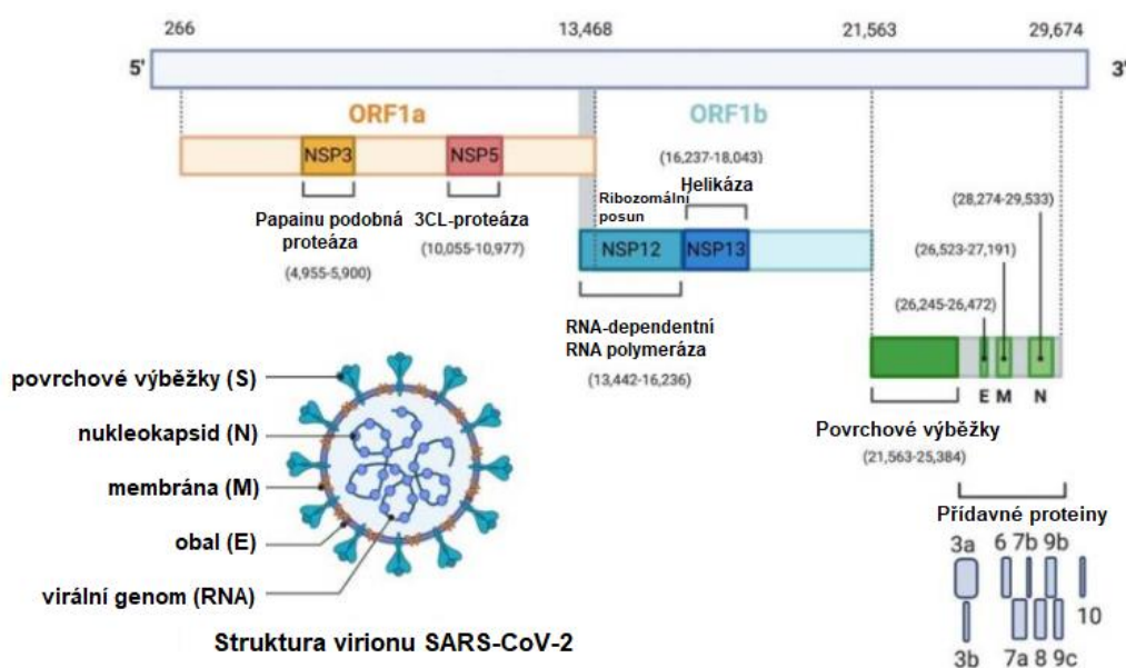
Obr. 3: Organizace genomu SARS-CoV-2 a struktura SARS-CoV-2 virionu (převzato: Alanagreh et al. , 2020, upraveno). Legenda: Genom SARS-CoV-2 kóduje dva velké čtecí rámce ORF1a (oranžově), ORF1b (modře), které kódují pro 15 nestrukturních proteinů. Genom také kóduje pro čtyři strukturální proteiny (zeleně) S (výběžky), E (obal), M (membrána) a N (nukleokapsid) a přidavné proteiny (šedě).
