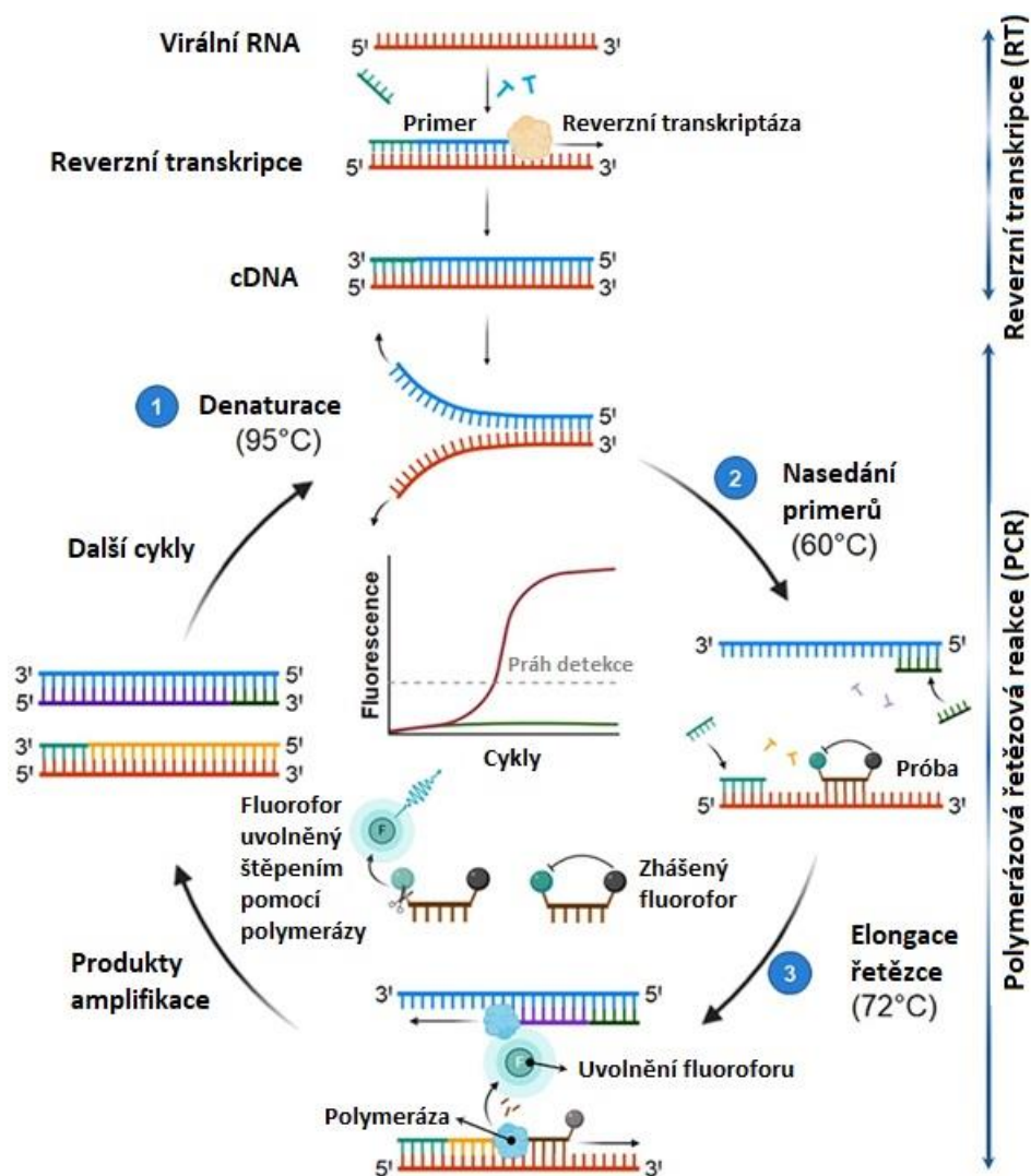
Obr. 6: Obecný princip polymerázové řetězové reakce s reverzní transkripcí v reálném čase (real-time RT-PCR). Legenda: Templát (virální RNA) je reverzní transkripcí přepsán do cDNA. Získaná cDNA je amplifikovaná pomocí PCR ve třech krocích: (1) denaturace cDNA, (2) nasednutí komplementárních primerů, (3) prodloužení řetězce pomocí enzymu DNA polymerázy. PCR je několikrát opakovaná, aby došlo k získání velkého množství amplikonů. Přítomnost cílových sekvencí je potvrzena fluorescenčním signálem, získaným ze sekvenčně specifických sond (převzato z Afzal , 2020, upraveno).
