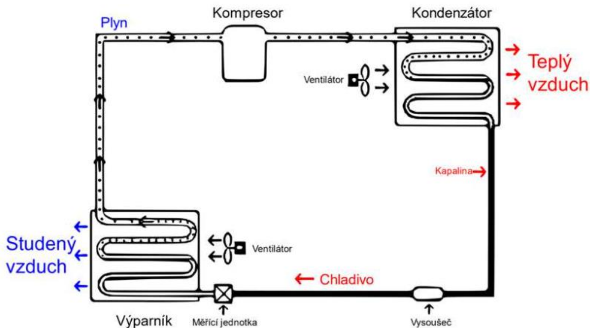
Obr. 2.1 Schéma klimatizace [7].
