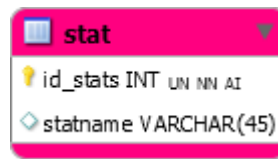
Obrázek 7: stat – tabulka v databázi (vlastní zpracování)
