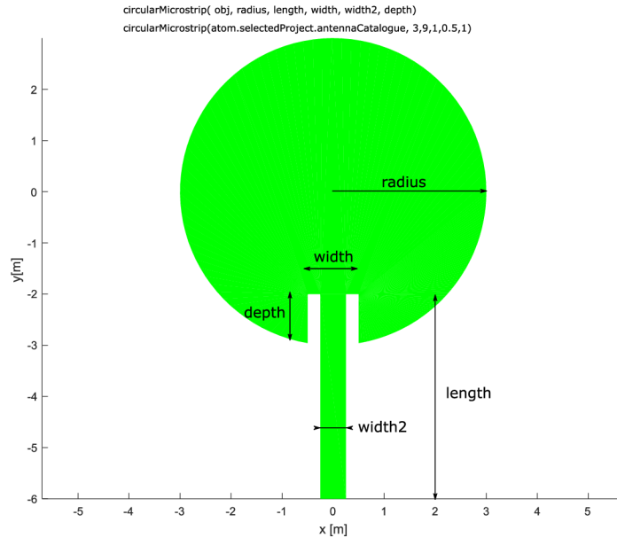
Obrázek 4.2.12 Vykreslení kruhového mikropásku po zavolení funkce circularMicrostrip.m .
