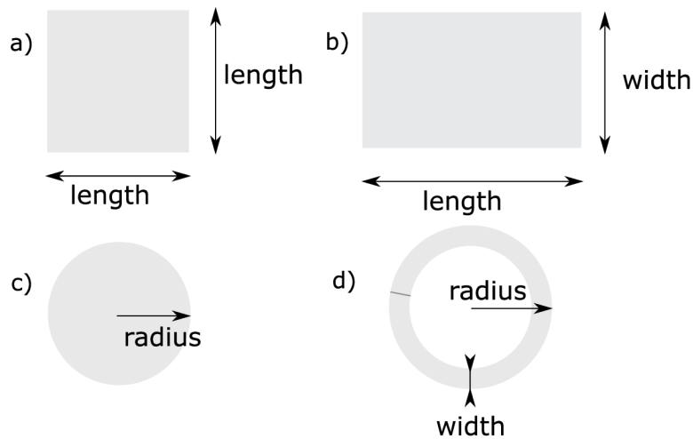
Obrázek 1.3.1 Příklady a) čtvercového, b) obdelníkového, c) kruhového, d) kružnicového tvaru s popisem rozměrů pro fličkovou anténu
