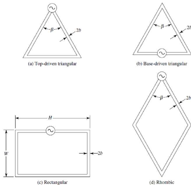
Obrázek 1.1.6 Základní tvary polygonálních smyčkových antén: trojúhelník (a, b), obdélník (c), kosodélník (d) [1]
