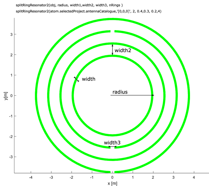
Obrázek 4.2.13 Vykreslení prstencového dutinového rezonátoru po zavolání funkce splitRingResonator2.m
