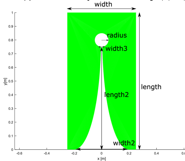
Obrázek 4.2.16 Vykreslení Vivaldiho antény po zavolání funkce vivaldiMicrostrip.m
