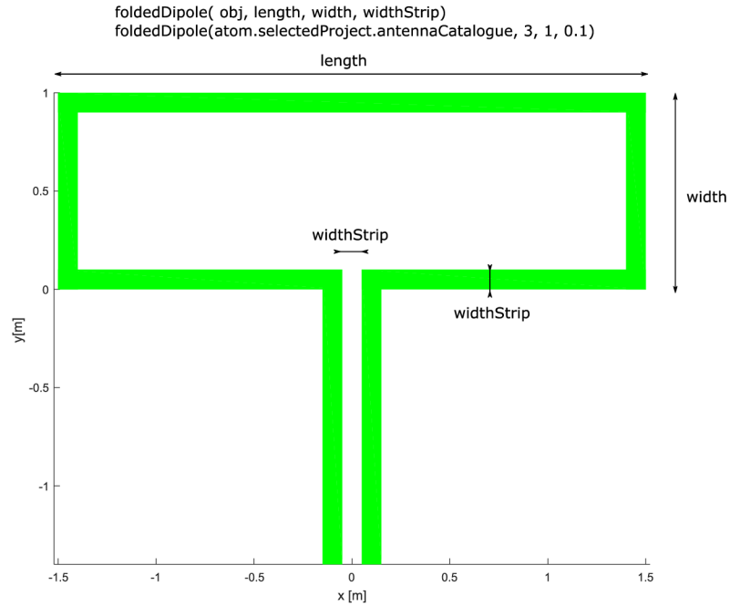
Obrázek 4.2.19 Vykreslení skládaného dipólu po zavolání funkce foldedDipole.m
