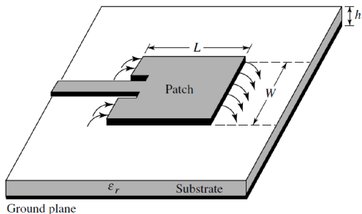
Obrázek 1.3.2 Ukázka tvaru a rozměrů obdelníkové fličkové antény [1].
