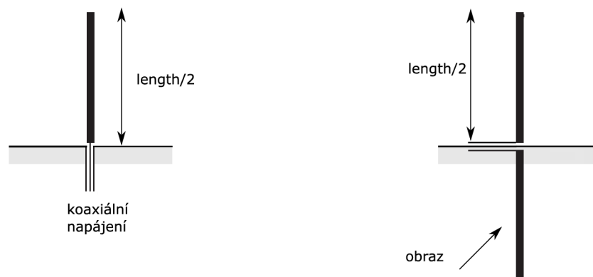
Obrázek 1.1.3 Čtvrtvlnný monopól nad zemní deskou a k němu ekvivalentní půlvlnný dipól [2]
