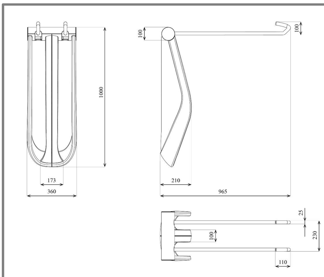
Obr. 5-8 Základní rozměry
