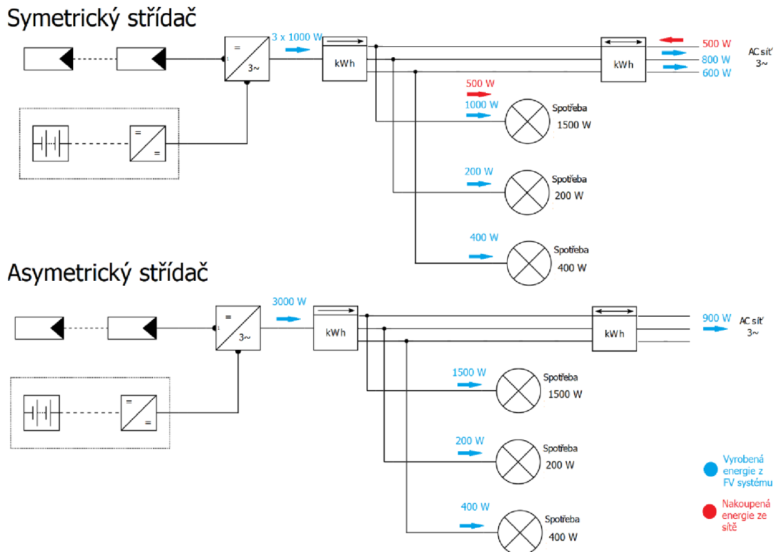
Obr. 5.2 Rozdíl mezi symetrickým a asymetrickým střídačem
