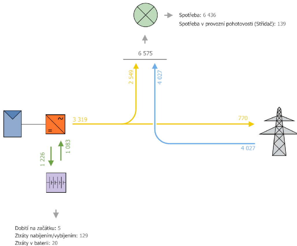
Obr. 8.8 Grafika toku energie FVS POLY
