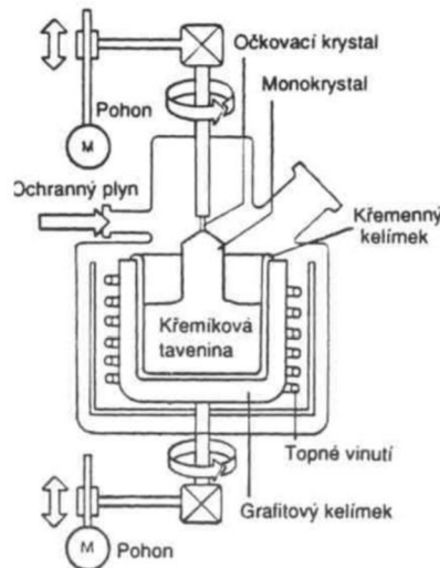
Obr. 3.1 Schematické znázornění výroby monokrystalu Czochralského metodou [6]
