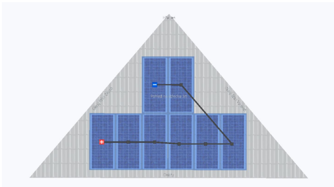
Obr. 8.7 Zapojení FVS POLY do série
