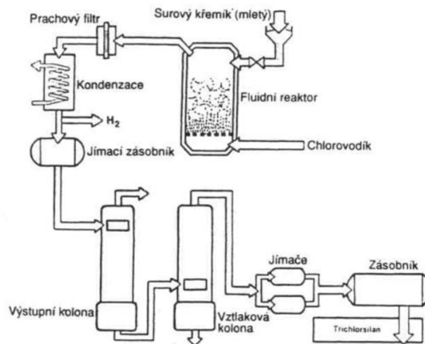
Obr. 3.3 Schéma syntézy trichlorsilanu a čistění pomocí destilace [6]
