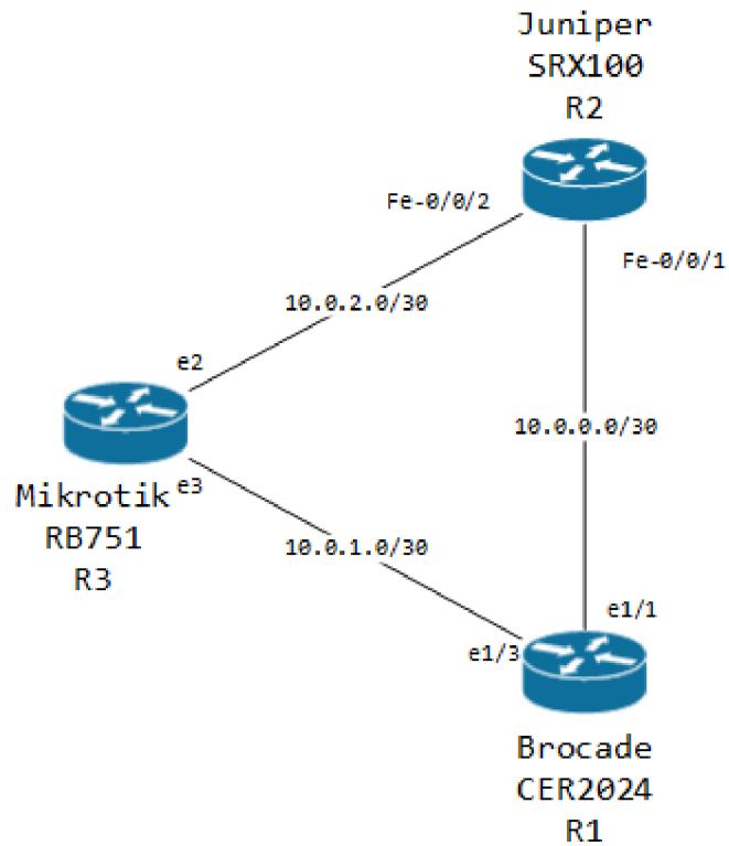
Obr. 3.1: Zapojení topologie.
