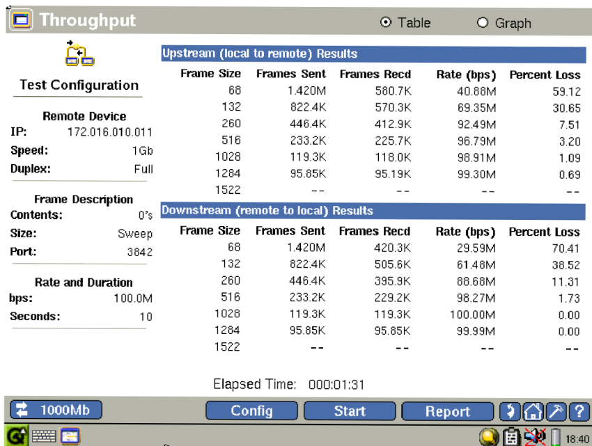
Obr. 3.5: Test propustnosti.
