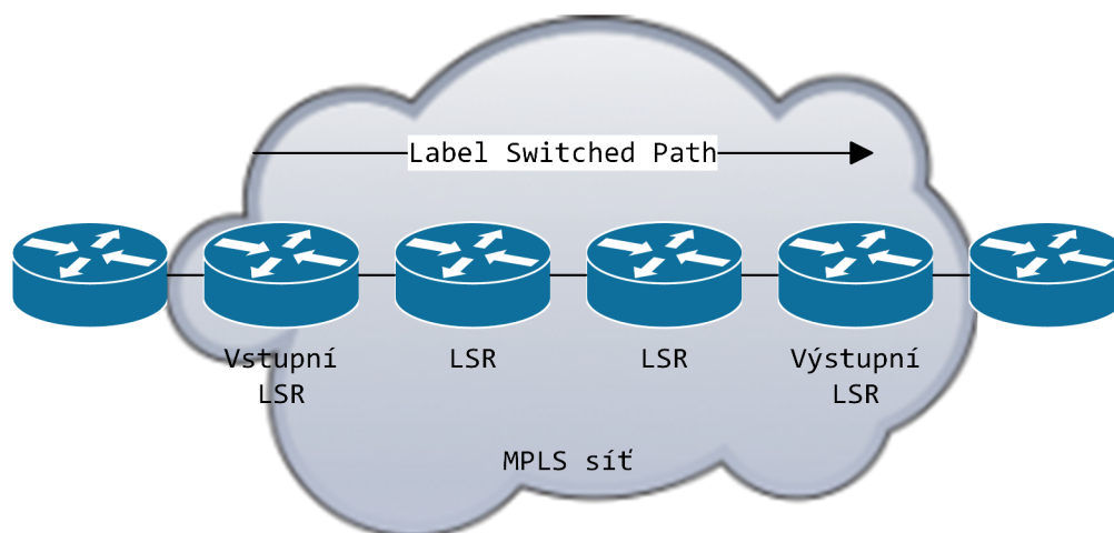
Obr. 1.3: MPLS síť.
